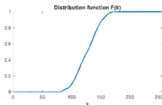
F1
