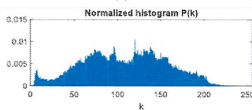
H1
