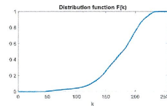
F3
